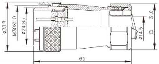
PLS-28-GPM4 4=轉接1/2"軟管
